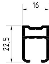
AL-IS.2 Führung „U“ Art.-Nr. 3003021FF
