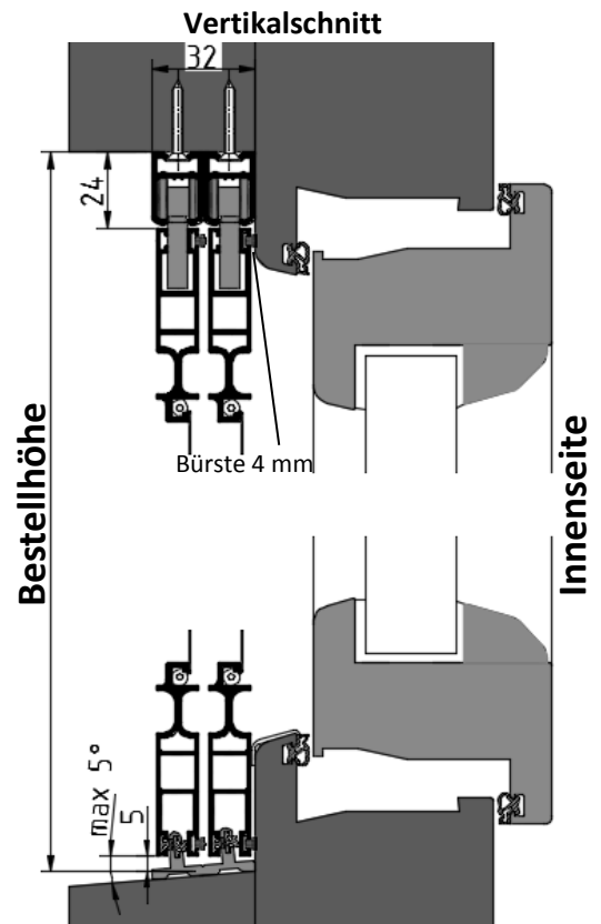
AL-IS.2 Führung „U“ Art.-Nr. 3003021FF
