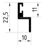
AL-IS.2 Z-Profil Art.-Nr. 3003022FF
