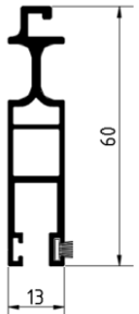
AL-IS.3 Flügelprofil ST mit Bürste 4mm / 20mm Art.-Nr. 3003016FF
