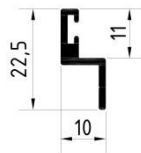
AL-IS.2 Z-Profil Art.-Nr. 3003022FF
