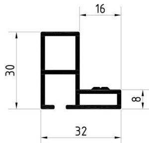
AL-IS.2 Rahmenprofil ST Art.-Nr. 3003010FF
