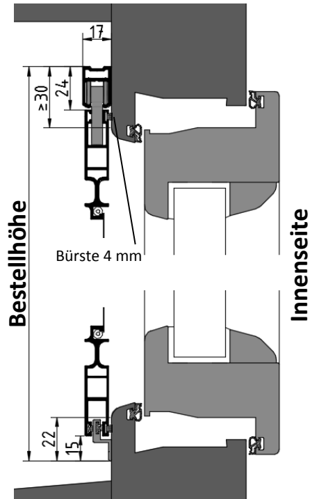
V1: Z-Schiene
