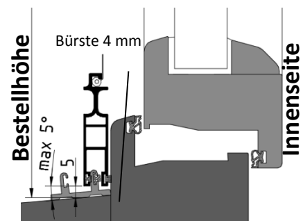
V2: Bodenschiene
