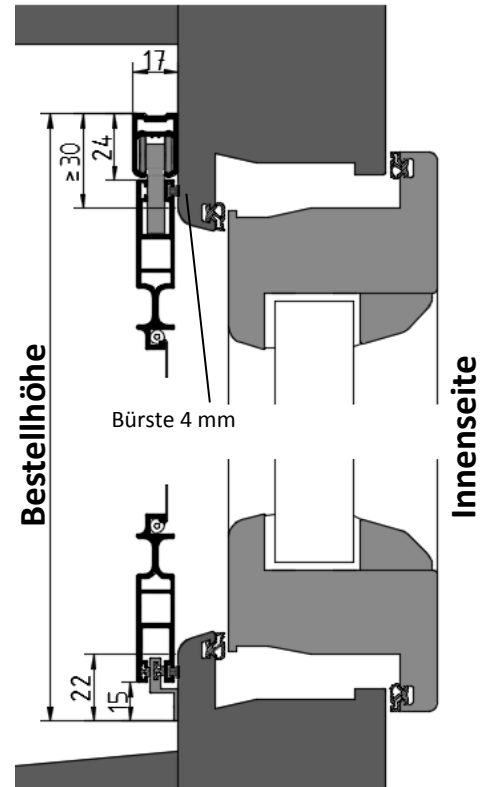
V1: Z-Schiene
