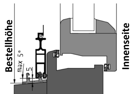
V2: Bodenschiene
